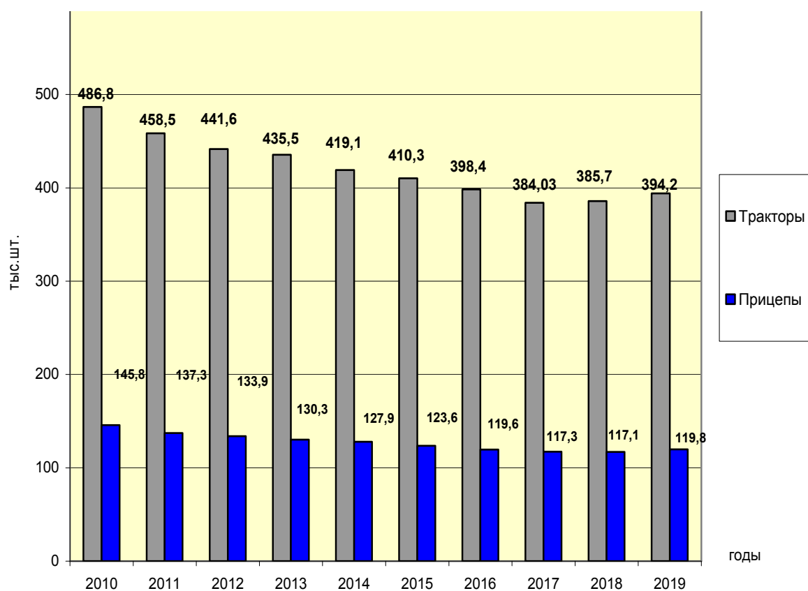
Рисунок 10 - Количество зарегистрированных прицепов и тракторов в АПК
