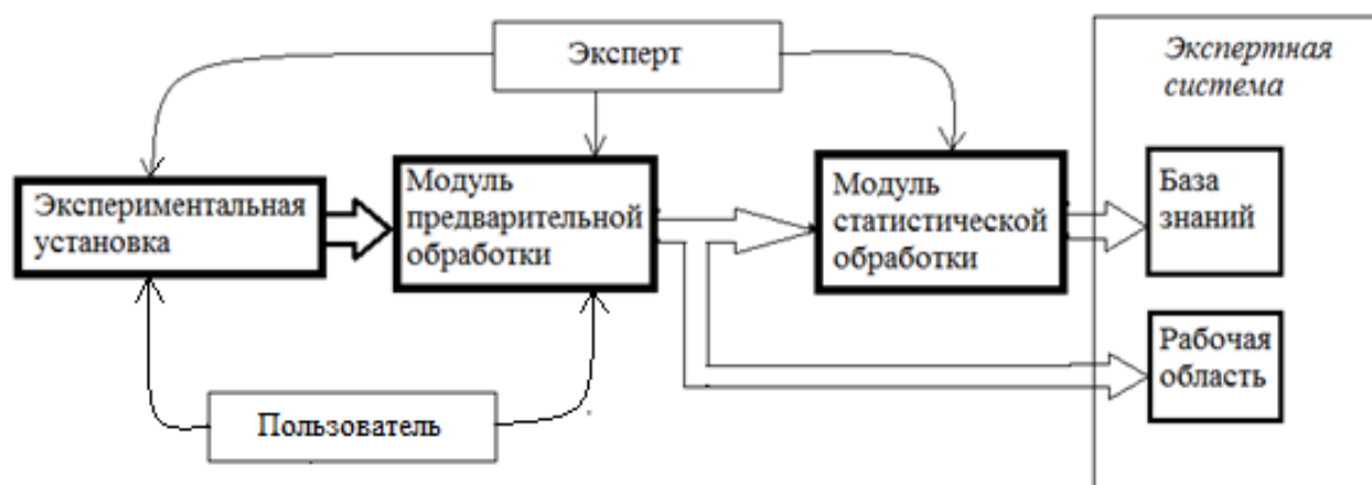
Рисунок 1 - Архитектура аппаратно-программного комплекса для формирования данных для экспертной системы
